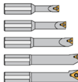
Utensili per testine di alesatura
